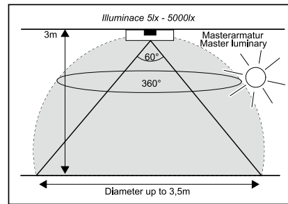
Detekteringsområde ljussensor
