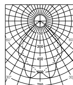
Bredstrålande med lamellbländskydd
